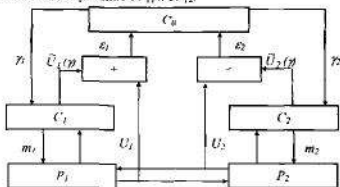
Рисунок 6.4 Двухуровневая система координации
