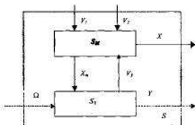
Рисунок 12.3 Связи управляющей системы S_M с внешней средой и объектом управления S_0
