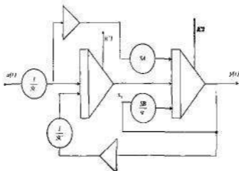
Рисунок 13.14 Аналоговая модель контура регулирования
