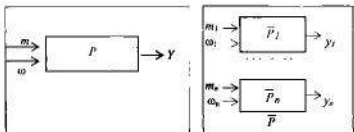
а) исходный управляемый процесс P б) процесс \bar{P} , полученный путем декомпозиции P на подпроцессы P_1, P_2, \dots, P_n
