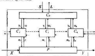
Рисунок 6.3 Двухуровневая иерархическая система управления
