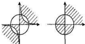
Рисунок 16.5 Допустимые множества
