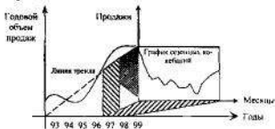
Рисунок 9.5 График тренда
