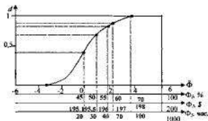
Рисунок 12.6 Функция желательности
