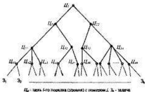
Рисунок 7.2 Дерево целей
