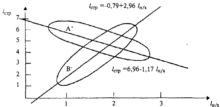
Рис. 37. Зависимость между трудовыми ресурсами в строительстве ( l_{стр} ) и в народном хозяйстве ( l_{н/х} ) в погодных темпах прироста в периоды А и В
